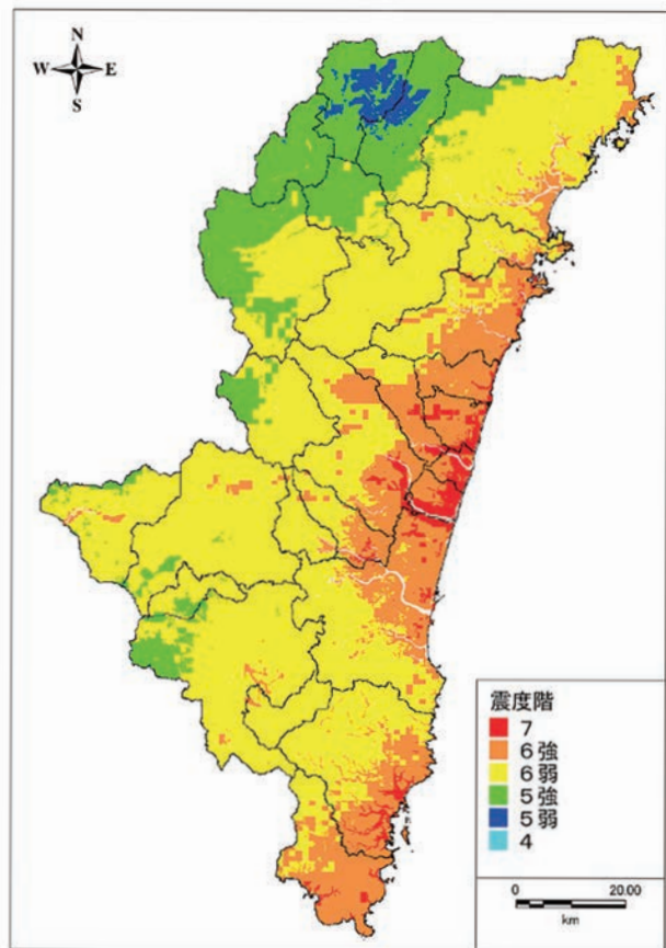
■図 地震動想定（震度分布） （「宮崎県地震・津波及び被害の想定について」令和2年3月より）
